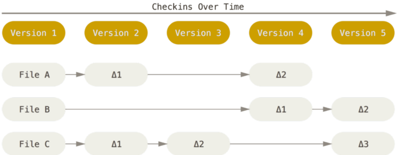
Figura 4. Memorizzazione dei dati come cambiamenti di ogni file da una versione di base.
