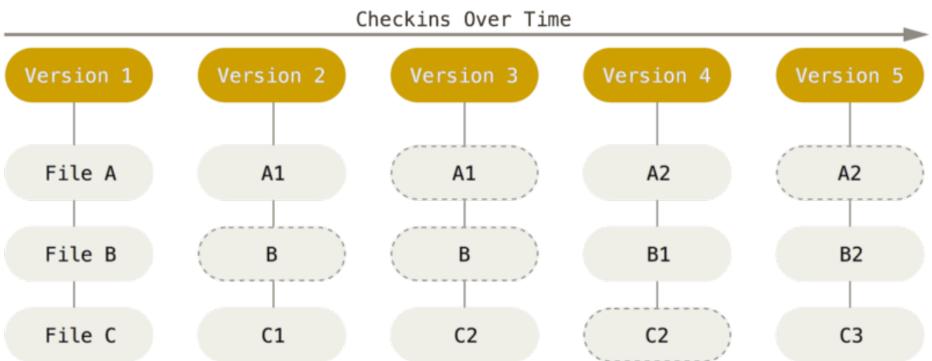
Figura 5. Memorizzazione dei dati come snapshot del progetto nel tempo.
