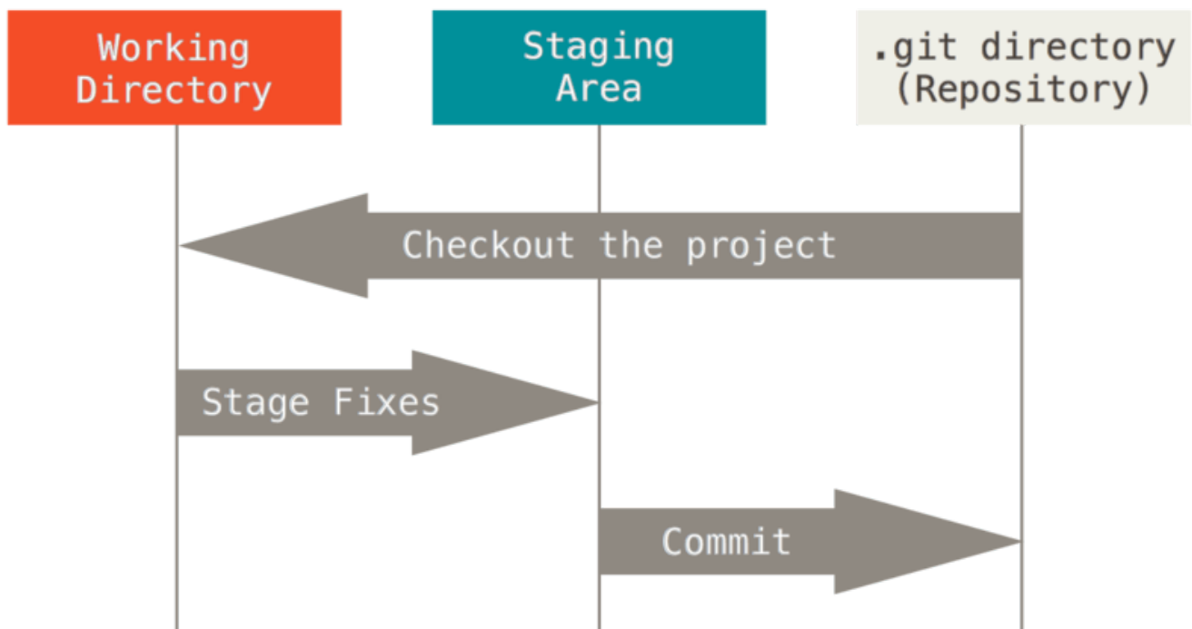
Figura 6. Albero di lavoro, area di stage e directory di Git.
