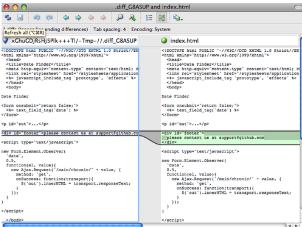
Figuur 143. P4Merge.
