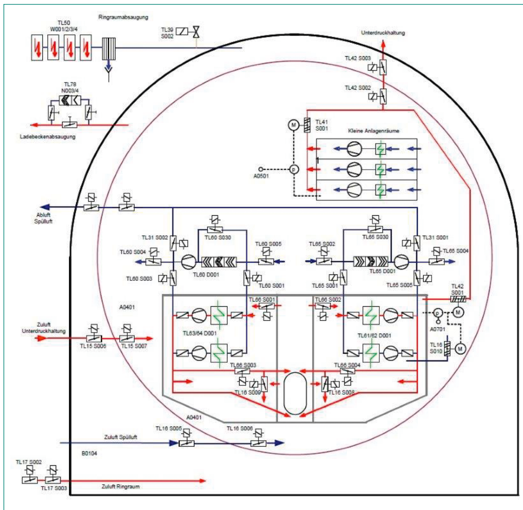
Abbildung 3: Kernkraftwerk Gösgen: Umluftkühlanlagen im Reaktorsicherheitsbe- hälter. Quelle: KKG EDMS: 559682 – Tech- nologiekurs
