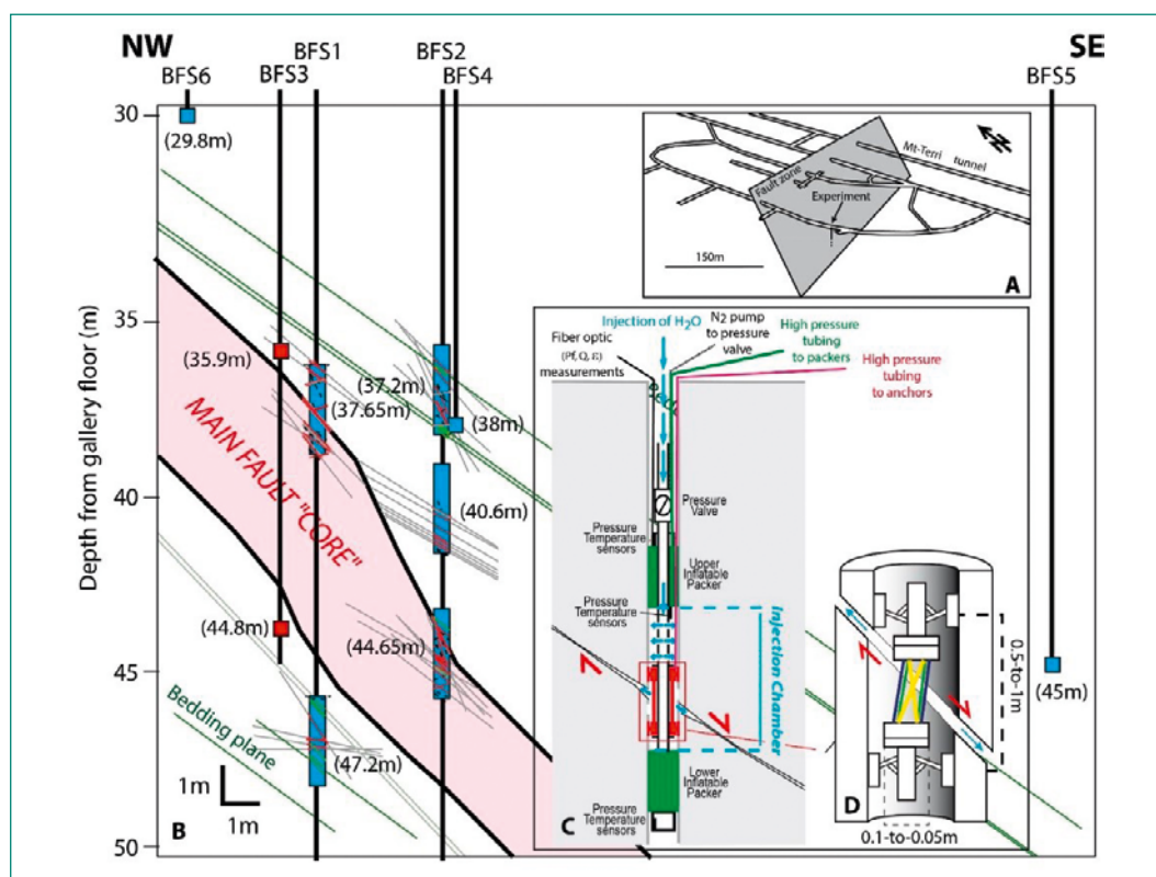
Abbildung 52: (A) 3D-Ansicht der Hauptstörung im Felslabor Mont Terri mit dem Ort des FS-Experiments; (B) Vereinfachter Schnitt durch die Hauptstörung mit der Position der Testintervalle (blaue Rechtecke) in den Bohrungen BFS-1 und BFS-2. In Bohrung BFS-3 erfolgt das passive seismische Monitoring; (C) Darstellung der SIMFIP Testausrüstung; (D) Schematische Darstellung der 3D-Deformationsmess Einheit. Quelle: «FS-Experiment»
