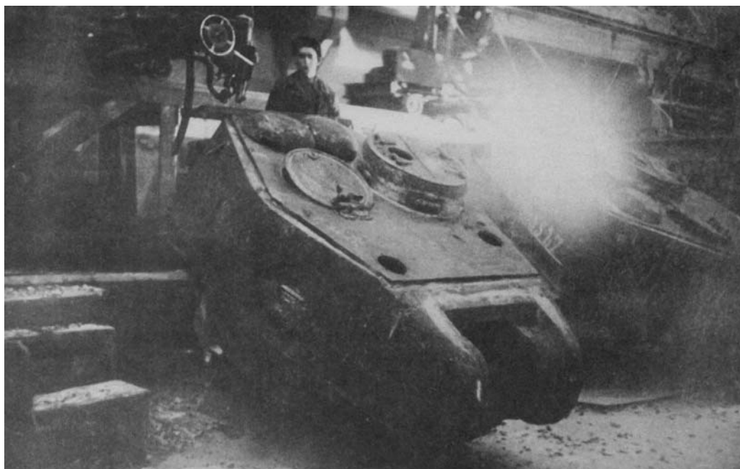
Автоматическая приварка крыши к литой бронебашне танка Т-34-85
