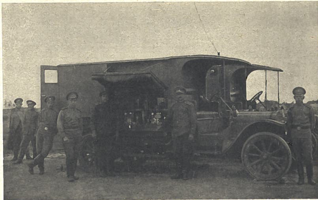
Машинная часть полевой радіо-станції.
