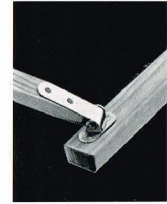
Ruderbeschläge.
