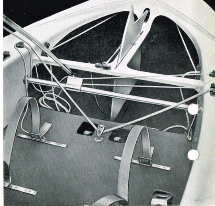
Alle Beschläge sind aus rostfreiem Stahl und Glasfaser, und das Schwert ist aus Aluminium.
