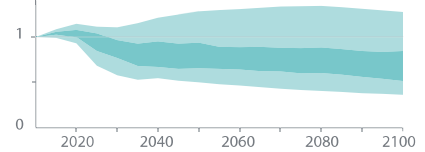
Net zero CO 2 도달 시기 선의 폭은 시나리오의 5-95분위와 25-75분위를 나타냄 오버슈트(overshoot)이 없거나 제한된 오버슈트 하에서 지구온난화를 1.5°C로 억제하는 경로 높은 오버슈트 하의 경로 지구온난화를 2°C 미만으로 억제하는 경로 (위에는 제시되지 않음)
