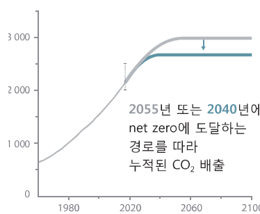
c) CO 2 순 누적 배출량
