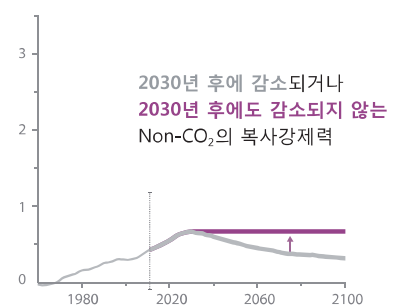
d) Non-CO 2 복사강제력 경로
