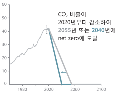
b) 모식화된 전지구 CO 2 순 배출 경로
