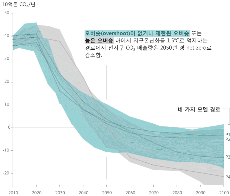
Net zero CO 2 도달 시기 선의 폭은 시나리오의 5-95분위와 25-75분위를 나타냄 오버슈트(overshoot)이 없거나 제한된 오버슈트 하에서 지구온난화를 1.5°C로 억제하는 경로 높은 오버슈트 하의 경로 지구온난화를 2°C 미만으로 억제하는 경로 (위에는 제시되지 않음)
