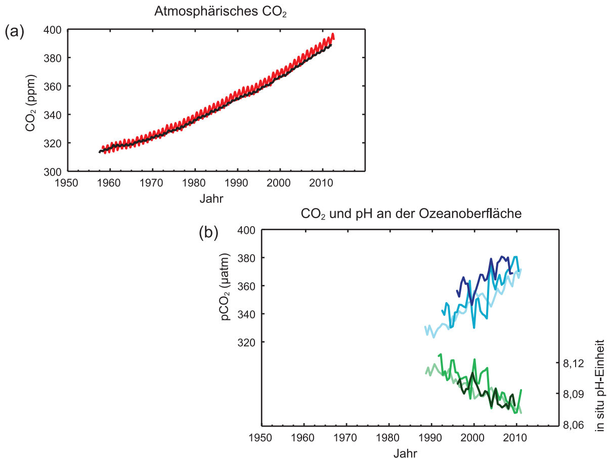
Abbildung SPM.4 | Mehrfache beobachtete Indikatoren eines sich verändernden globalen Kohlenstoffkreislaufs: (a) Atmosphärische Kohlendioxid (CO 2 )-Konzentrationen vom Mauna Loa (19°32'N, 155°34'W – rot) und vom Südpol (89°59'S, 24°48'W – schwarz) seit 1958. (b) Teildruck von gelöstem CO 2 an der Ozeanoberfläche (blaue Kurven) und in situ pH (grüne Kurven), ein Maß für den Säuregehalt des Ozeanwassers. Die Messungen stammen von drei Stationen aus dem Atlantik (29°10'N, 15°30'W – dunkelblau/dunkelgrün; 31°40'N, 64°10'W – blau/grün) und dem Pazifischen Ozean (22°45'N, 158°00'W – hellblau/hellgrün). Vollständige Einzelheiten der hier dargestellten Datensätze sind im zugrundeliegenden Bericht und im Zusatzmaterial zur Technischen Zusammenfassung zu finden. (Abbildungen 2.1 und 3.18; Abbildung TS.5)
