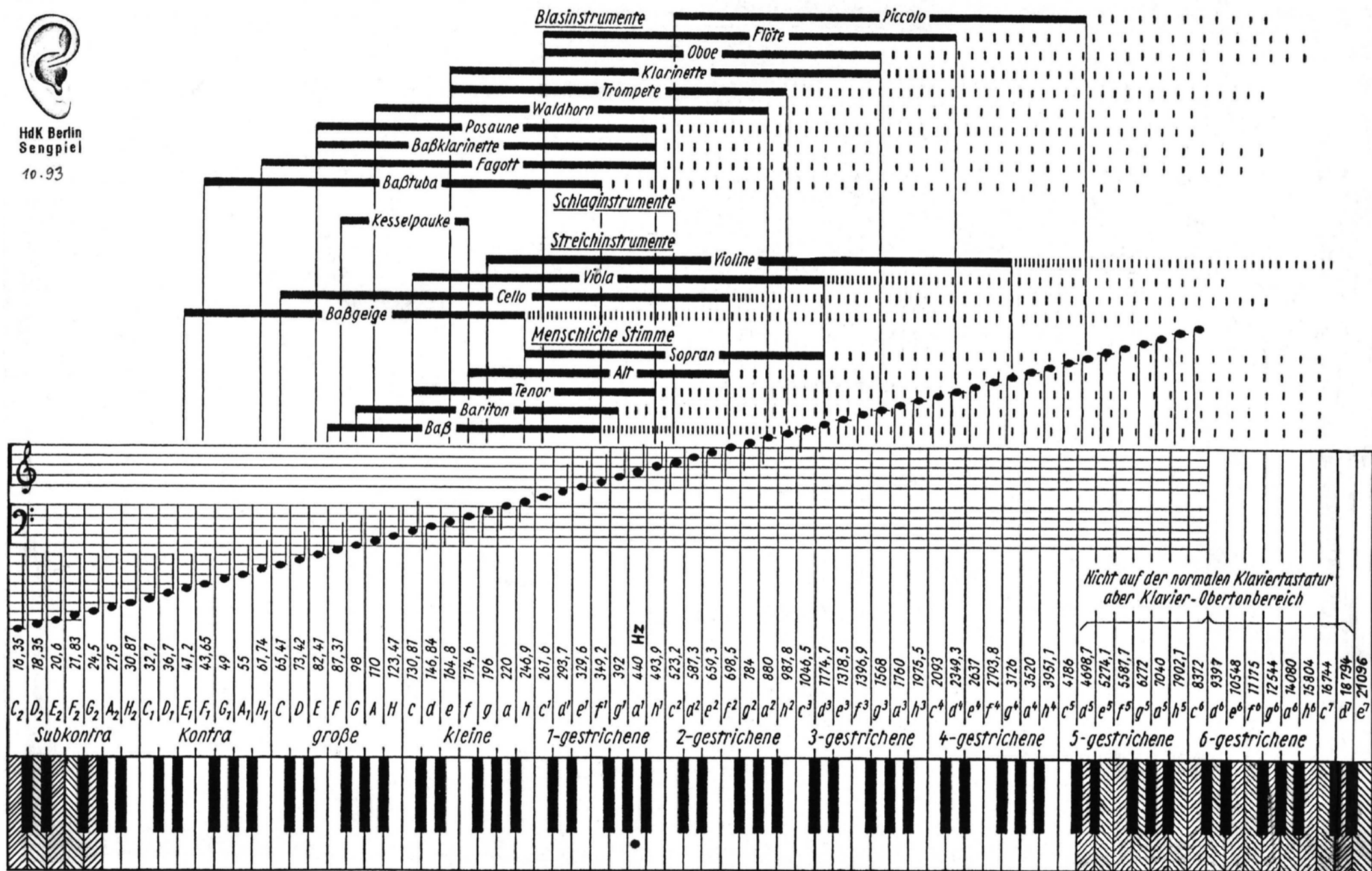
Frequenzbereich der Musikinstrumente und der Gesangsstimmen
