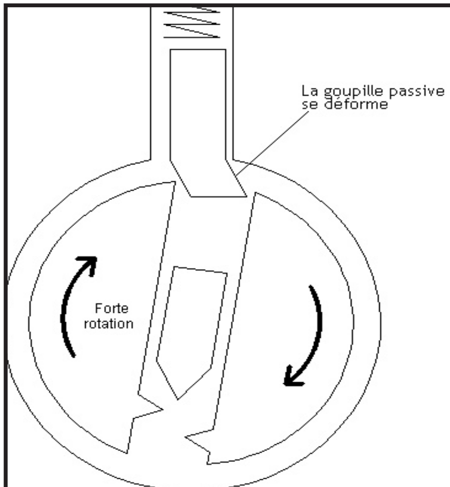
Schéma 9.2 : La goupille est faussement positionnée à cause des déformations dues à l'élasticité du matériau.
