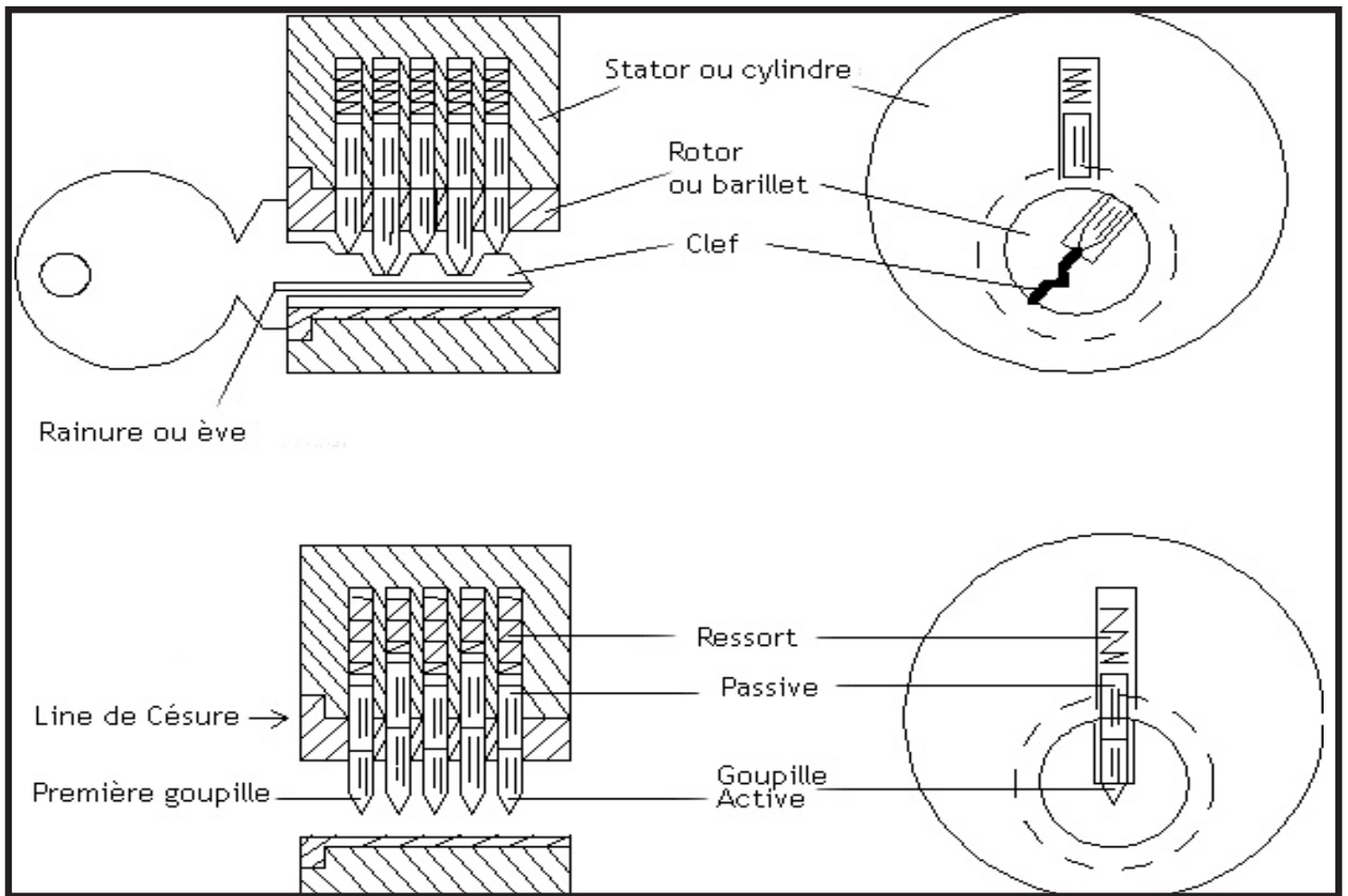
Schéma 2.1 : Fonctionnements des serrures à goupilles
