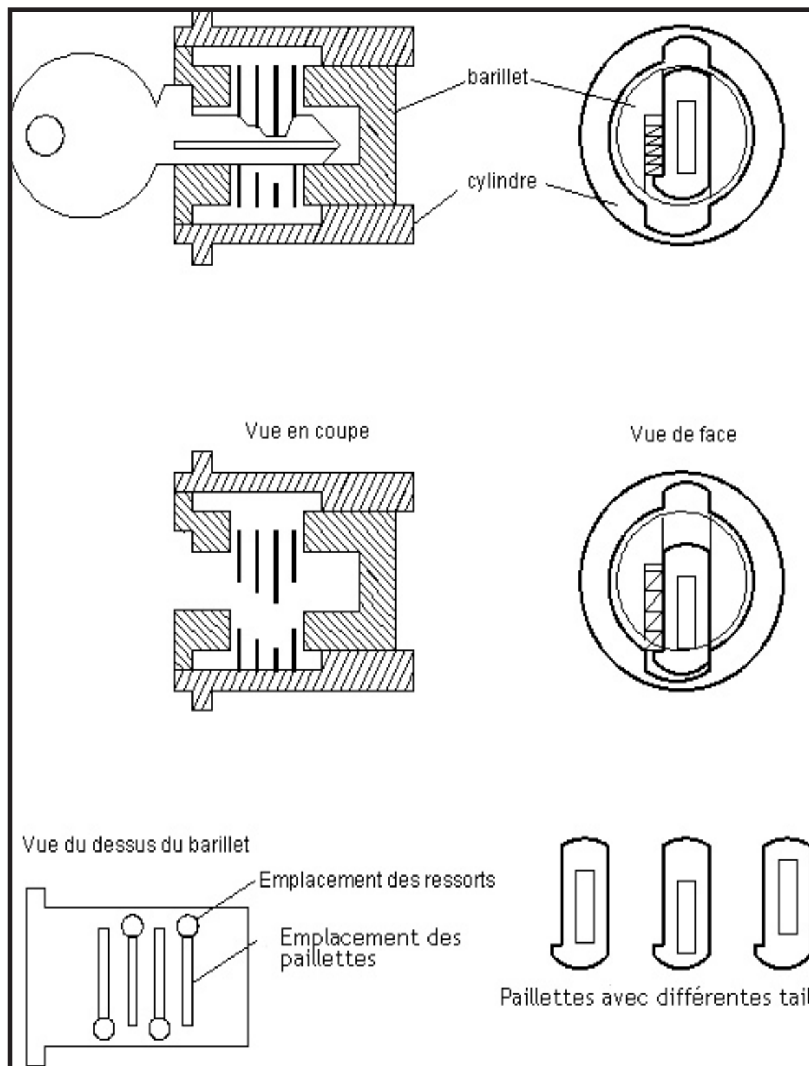
Schéma 9.10 : Fonctionnement d'une serrure à paillettes
