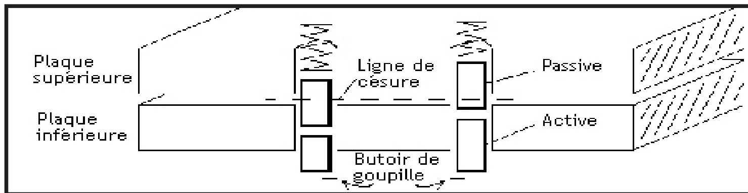
Schéma 3.1 : Modèle de serrure
