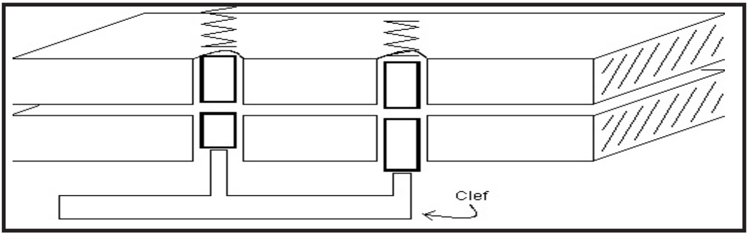
Schéma 3.2: (a) La clef lève les goupilles
