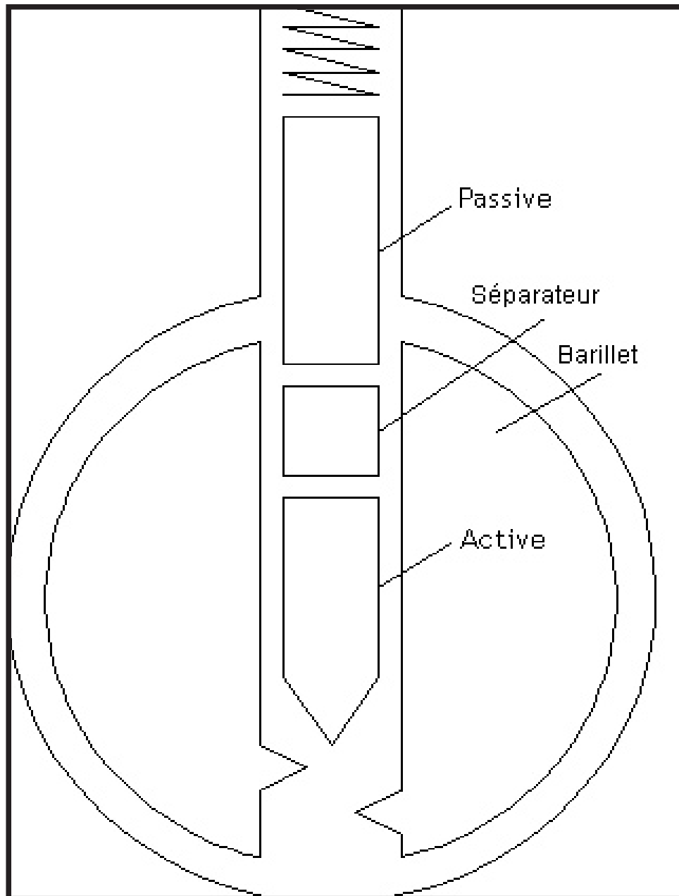
Schéma 9.8 : Séparateur pour clef «passe partout»
