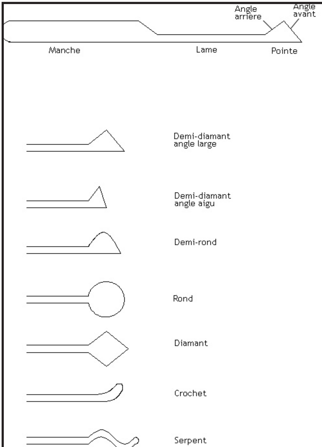
Schéma A.1: Différentes formes de crochets palpeurs
