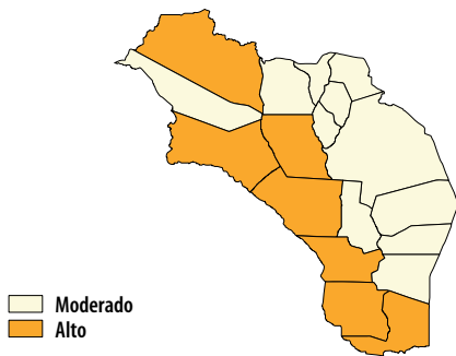
(1-3) Amenaza sísmica
