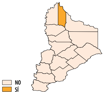
(1-3) Deslizamiento
