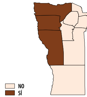
(1-2) Amenaza sísmica
