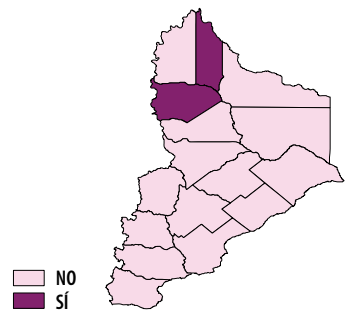
(1-4) Vulcanismo
