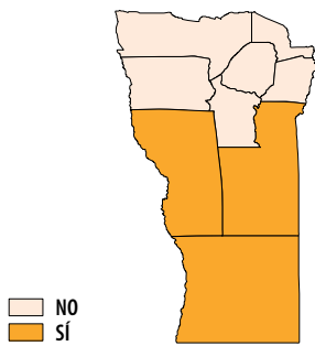
(1-3) Erosión Eólica
