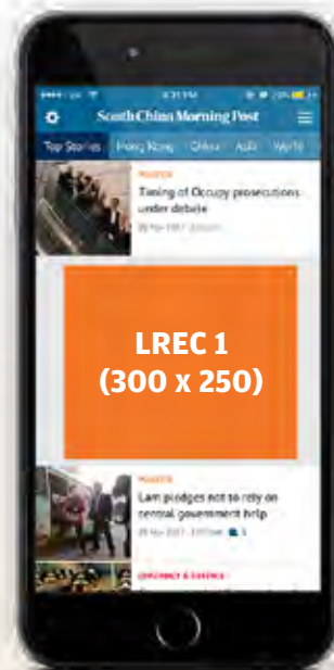
LREC 1
