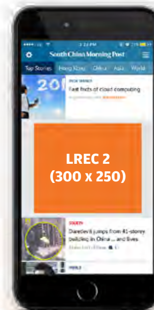
LREC 2
