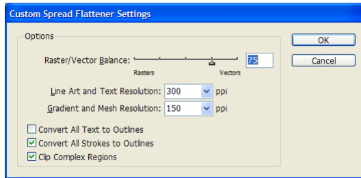
Figure 29. FlattenerPreference
