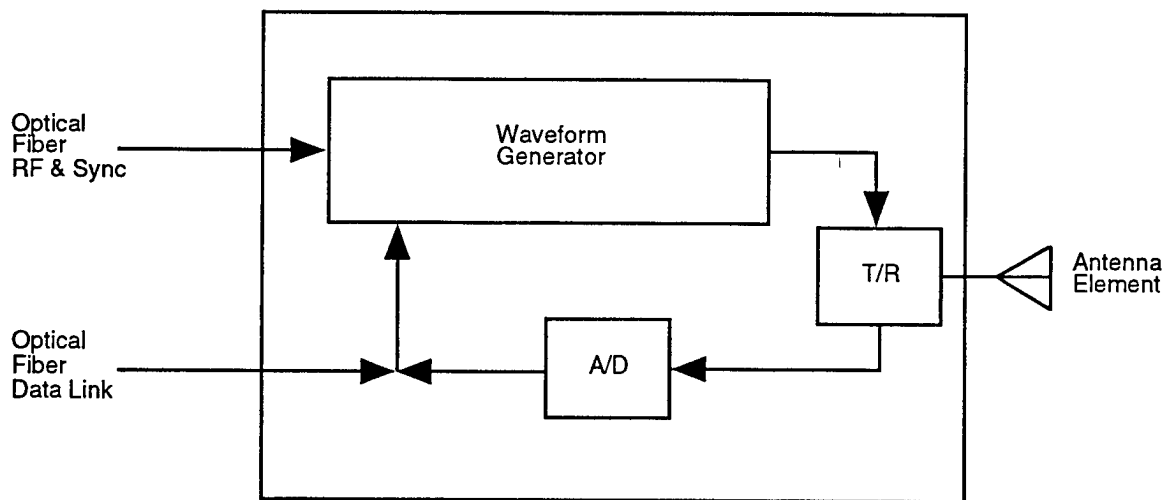
Figure 3-4. Array module.
