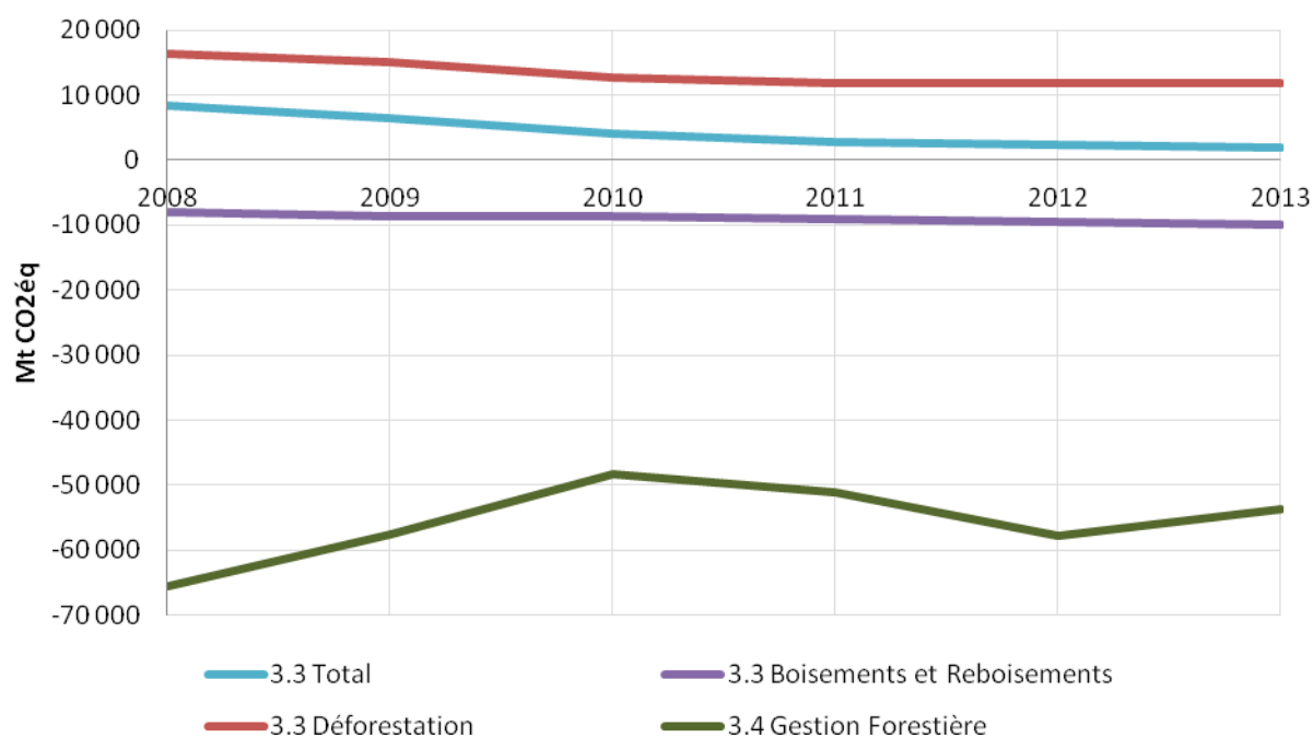
Figure 7.1 : Evolution des émissions / absorptions GES des activités du secteur UTCATF (format Kyoto, Inventaire v2015 pour l'année 2013)
