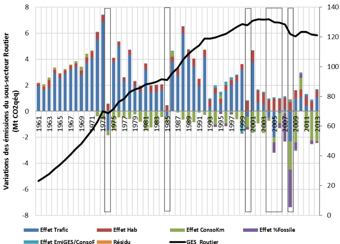
Figure 6.6 : variation des émissions du sous-secteur routier
