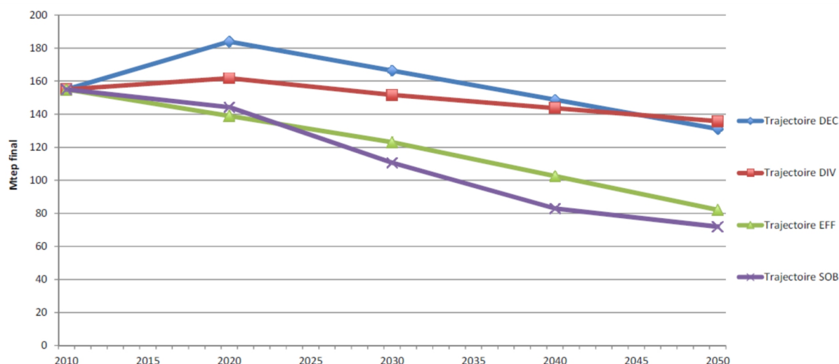
Figure 1.4 : Consommation finale énergétique selon les quatre « trajectoires DNTE » (source : groupe de travailGT2 « Scénarios et mix énergétique » du DNTE, juillet 2013)
