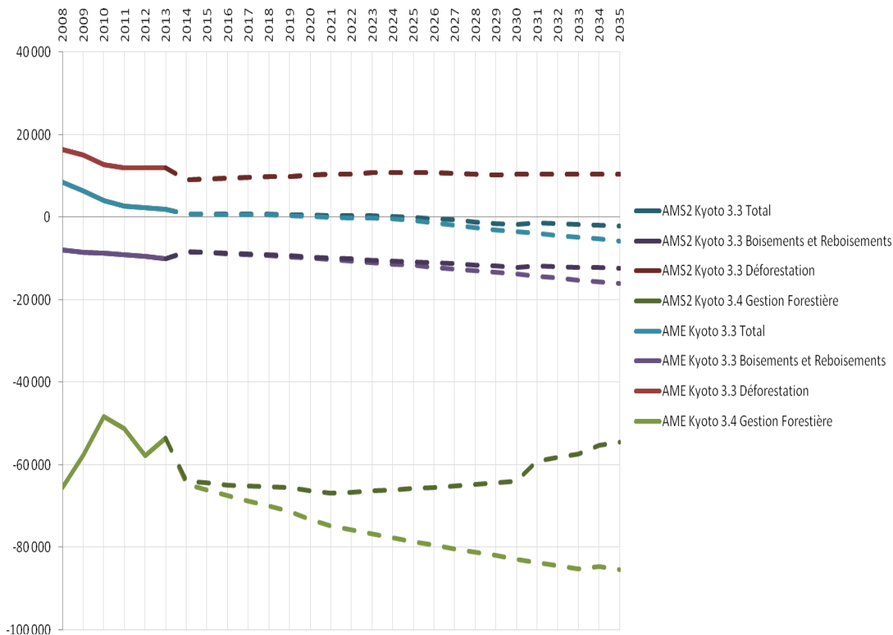
Figure 7.4 : Evolution des émissions / absorptions GES projetés des activités du secteur UTCF (format Kyoto, Scénarios prospectifs 2035 - Citepa) version 2 (traits en continu : inventaire 2013 v2015, format Kyoto ; traits discontinus : projection)
