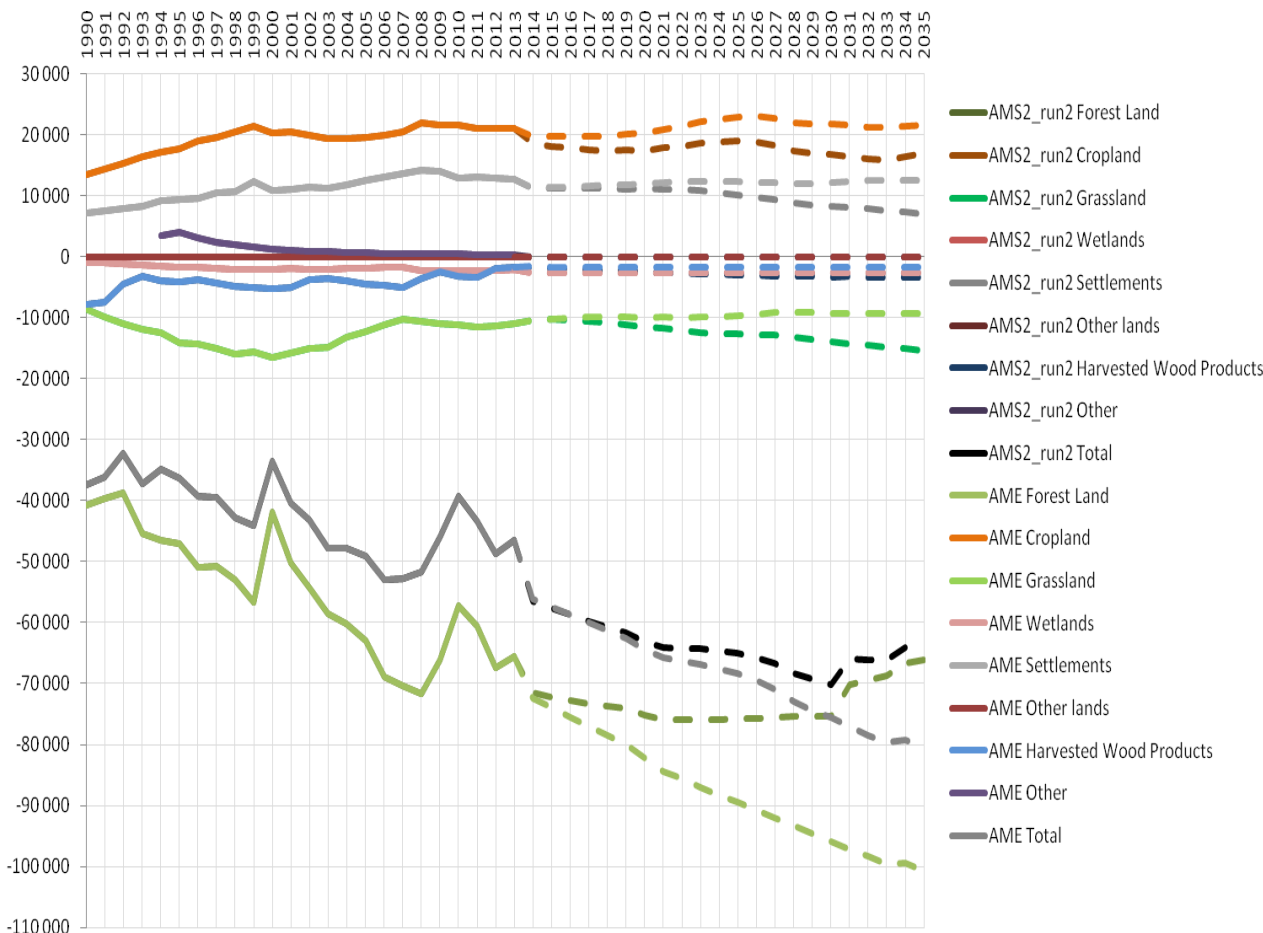
Figure 7.5 : Evolution des émissions / absorptions GES projetés des activités du secteur UTCF (format CCNUCC, Scénarios prospectifs 2035 - Citepa) version 2 (traits en continu : inventaire 2013 v2015, format Kyoto ; traits discontinus : projections)
