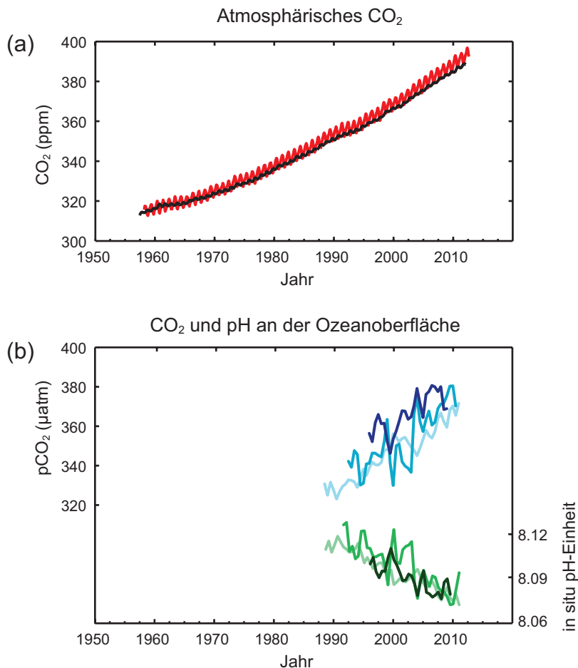
Abbildung SPM.4 | Mehrfache beobachtete Indikatoren eines sich verändernden globalen Kohlenstoff-Kreislaufs: (a) Atmosphärische Kohlendioxid (CO 2 )-Konzentrationen vom Mauna Loa (19°32'N, 155°34'W – rot) und vom Südpol (89°59'S, 24°48'W – schwarz) seit 1958. (b) Teildruck von gelöstem CO 2 an der Ozeanoberfläche (blaue Kurven) und in situ pH (grüne Kurven), ein Maß für den Säuregehalt des Ozeanwassers. Die Messungen stammen von drei Stationen aus dem Atlantik (29°10'N, 15°30'W – dunkelblau/dunkelgrün; 31°40'N, 64°10'W – blau/grün) und dem Pazifischen Ozean (22°45'N, 158°00'W – hellblau/hellgrün). Vollständige Einzelheiten der hier dargestellten Datensätze sind im zugrundeliegenden Bericht und im Zusatzmaterial zur Technischen Zusammenfassung zu finden. (Abbildungen 2.1 und 3.18; Abbildung TS.5)
