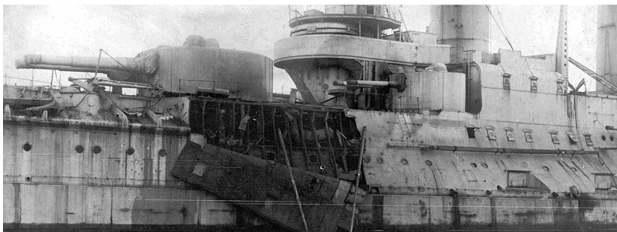
Poškozená sovětská bitevní loď Graždanin (bývalý Cesarevič), odstavená v roce 1921 v kronšadtském přístavu.
