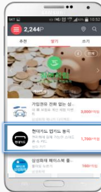
리워드오퍼월
