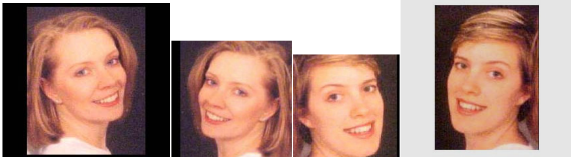
CNN
