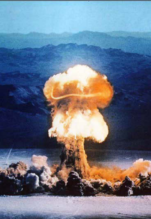
Bolet atòmic: explosió d'un dispositiu nuclear de 37 quilotones a Nevada. Crèdit: Govern dels Estats Units.
