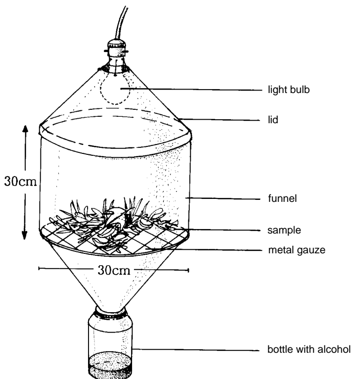
Fig. 55. Berlese (Tullgren) funnel
