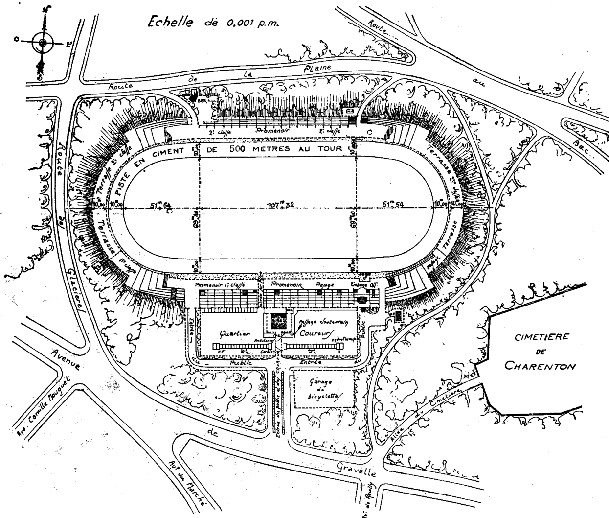
PLAN DU VÉLODROME MUNICIPAL DE VINCENNES.
