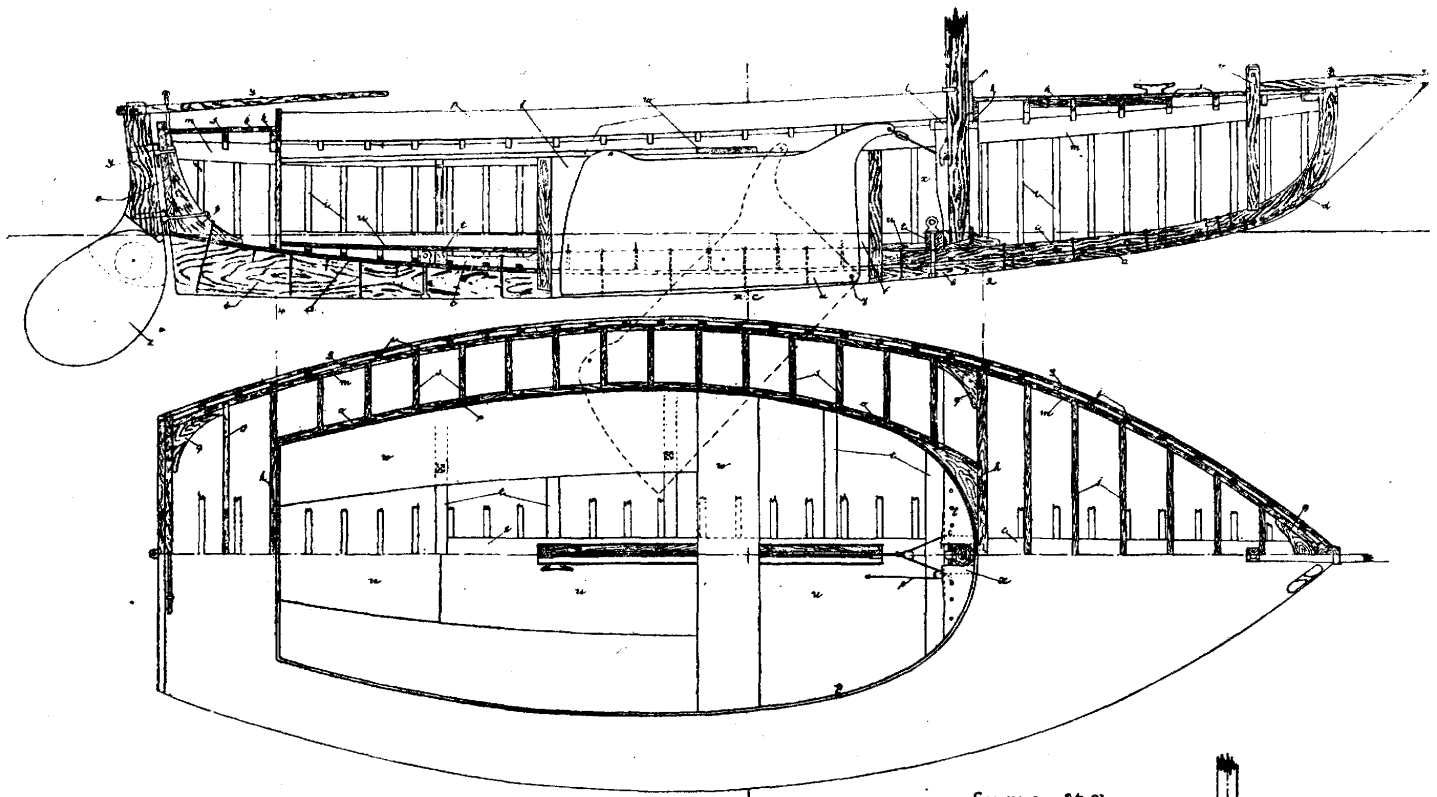
Plan des formes.
