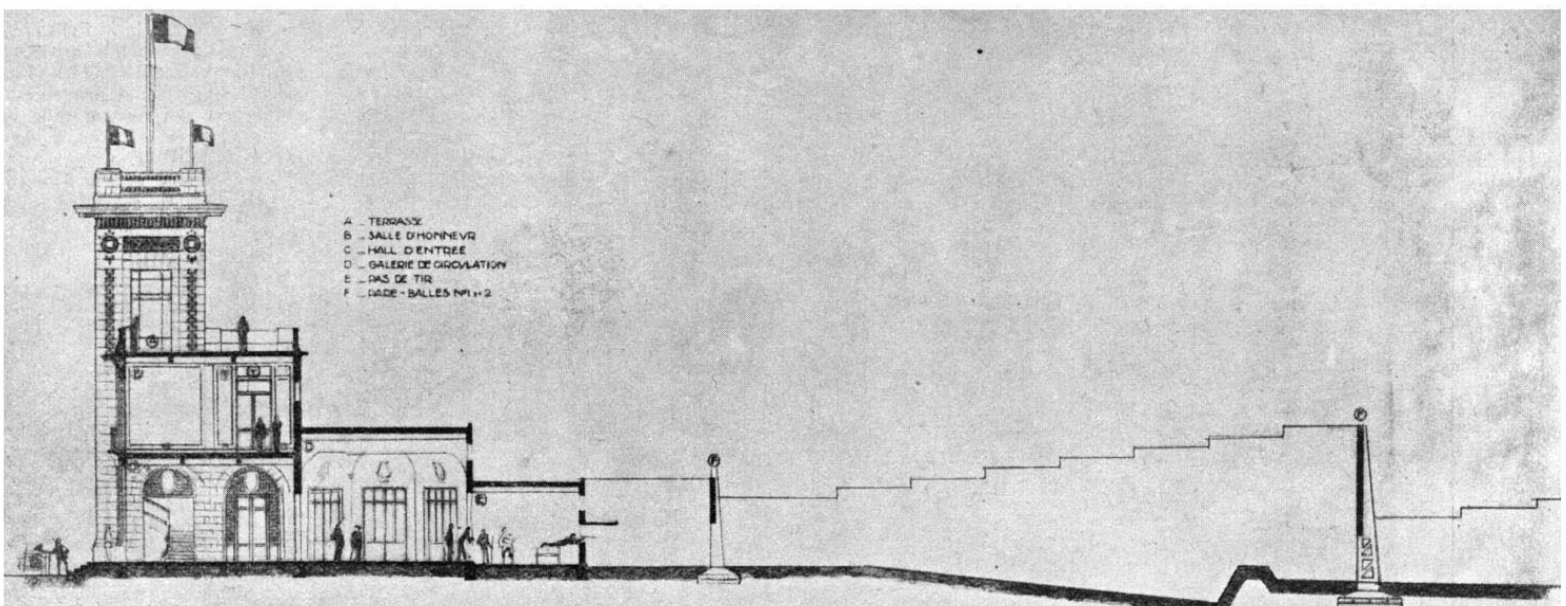
Coupe transversale.
