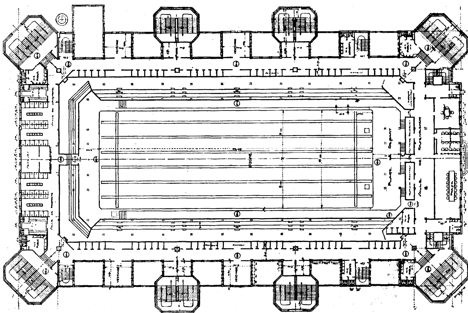
PLAN DU DEUXIÈME ÉTAGE
