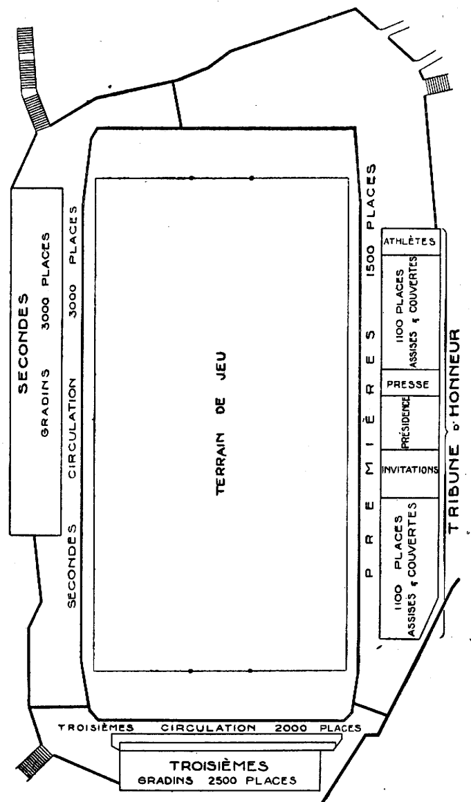
Dispositif des emplacements réservés aux spectateurs.
