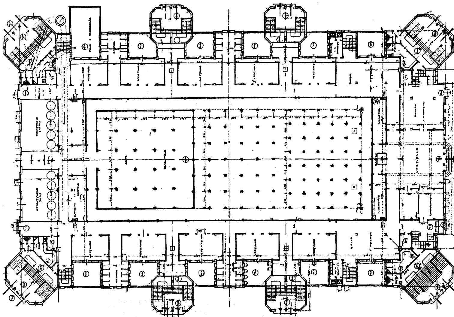
PLAN DU REZ-DE-CHAUSSÉE
