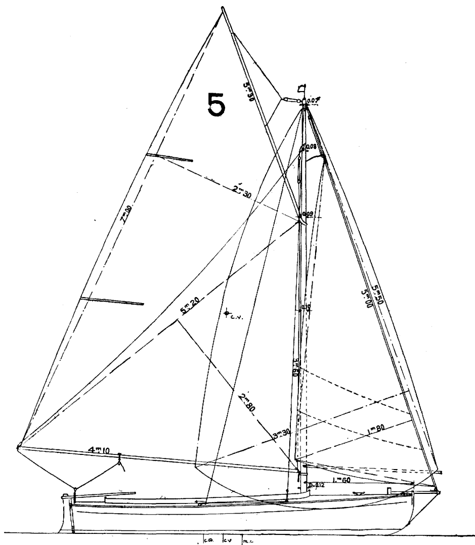
LE MONOTYPE OLYMPIQUE. — Plan de la voilure :
