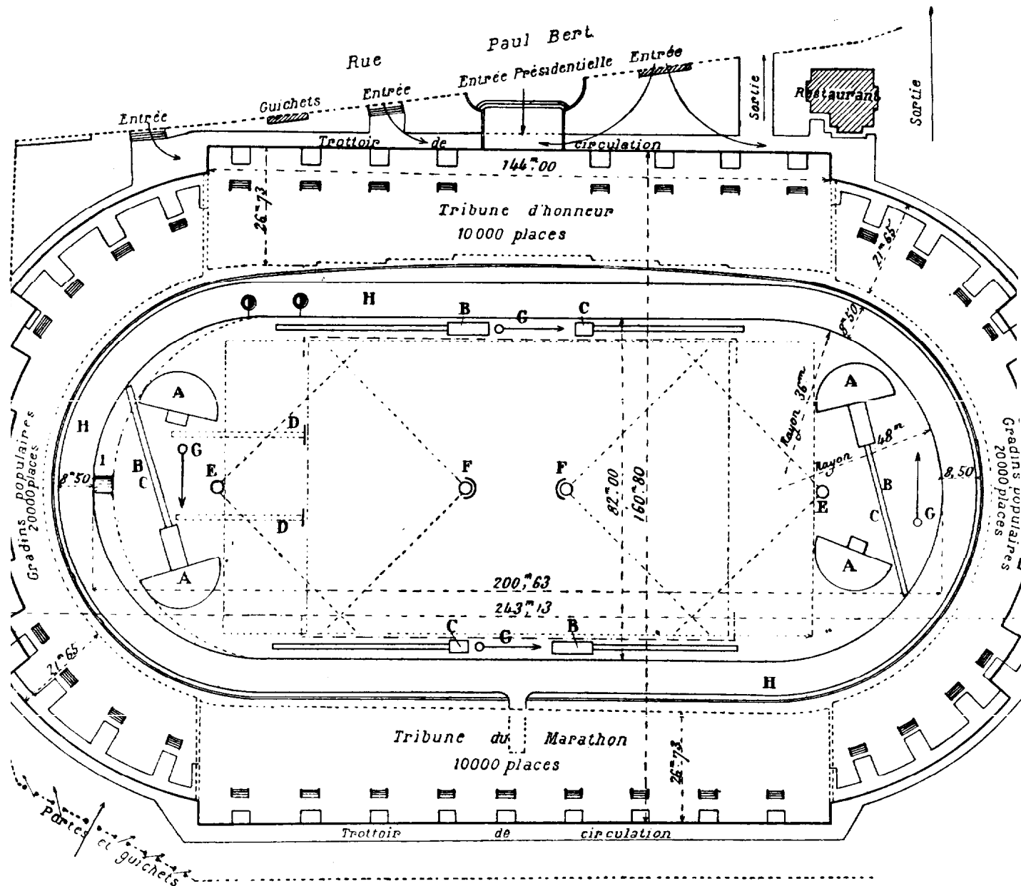
PLAN D'ENSEMBLE DU STADE OLYMPIQUE DE COLOMBES
