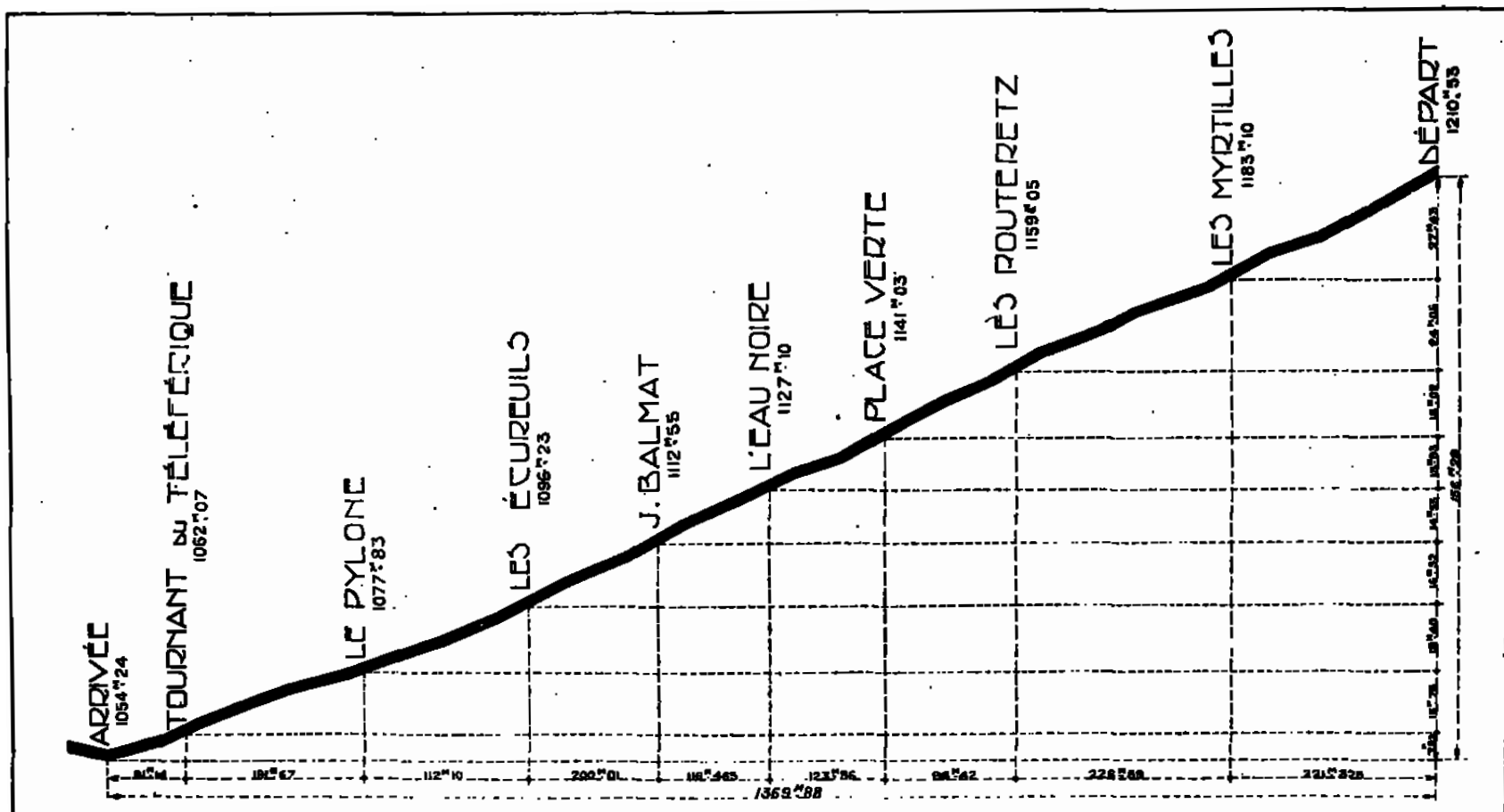
Profil.
