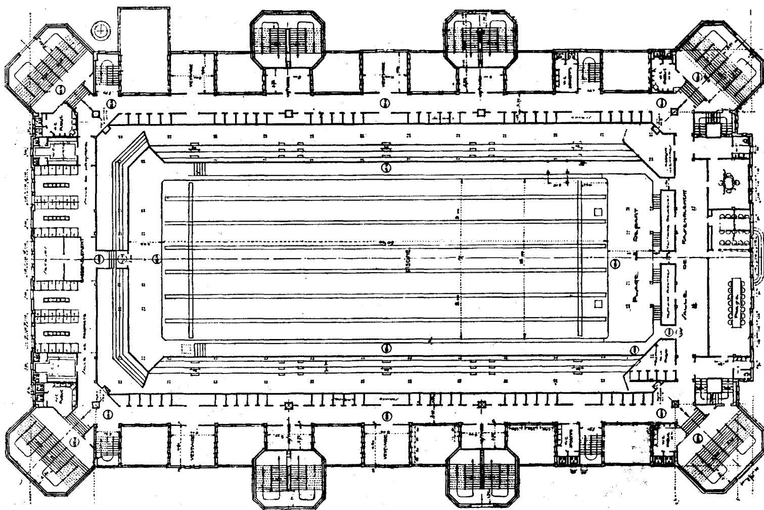
PLAN DU DEUXIÈME ÉTAGE
