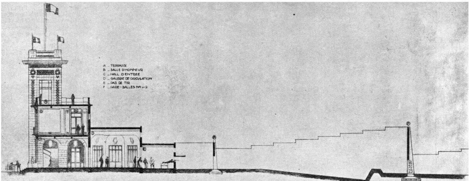
Coupe transversale.
